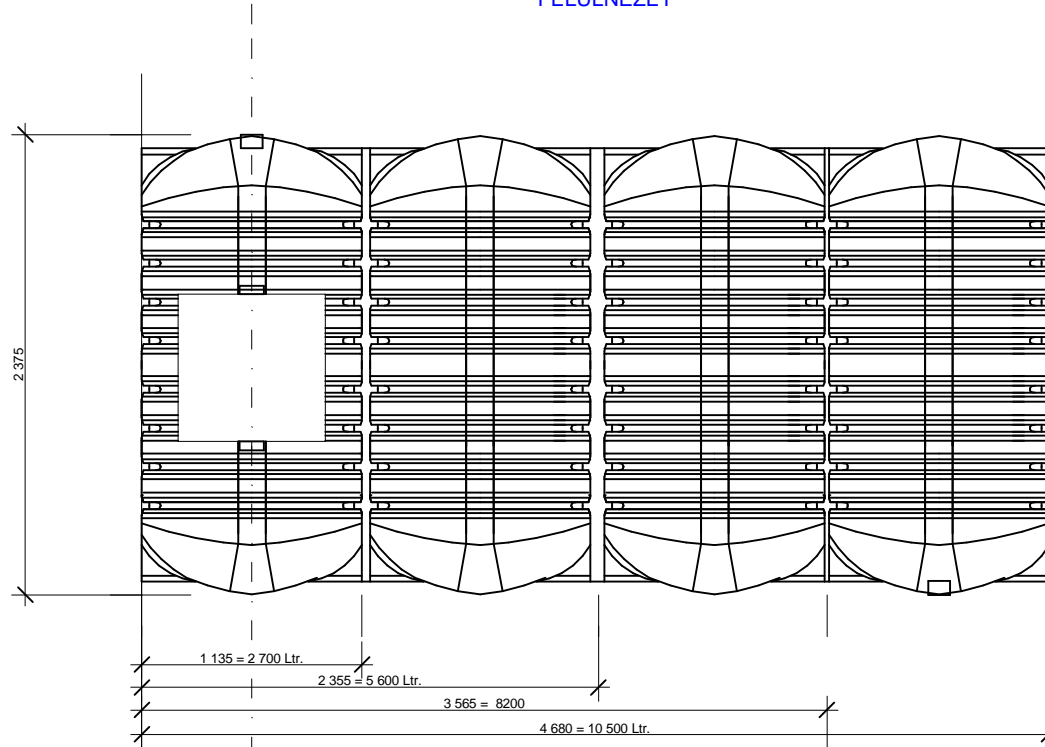
RIKUTEC AT 112 TARTÁLY FELÜLNÉZET
