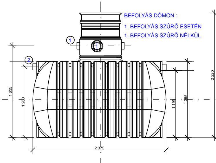
RIKUTEC AT 112 TARTÁLY OLDALNÉZET
