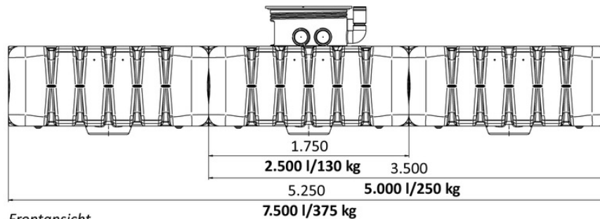
Frontansicht
